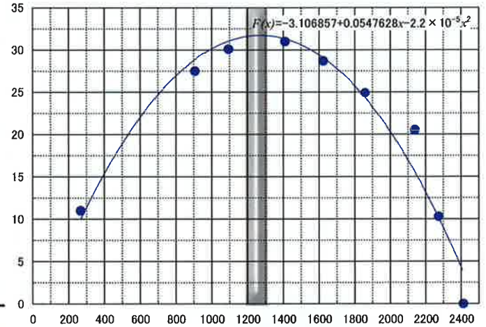
液体の圧力とモーター効率の関係(近似式)
